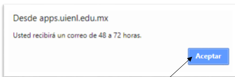
Figura 4 Mensaje
